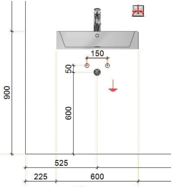
afvoer/toevoer wastafel
